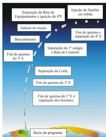
Figura 3: Perfil da missão do VLS-1 (AEB, 2007).
