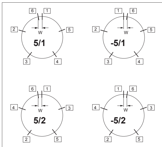
Figura 4: Seqüência dos pontos de partida de um ciclo para: número de padrão / índice de salto de 5/1, -5/1, 5/2, -5/2.
